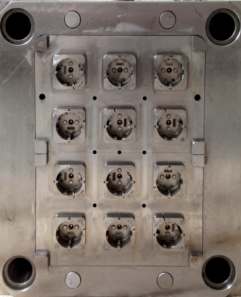
12-fach-Werkzeug für Steckdosen-Abdeckungen
