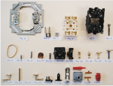
Aus diesen Einzelteilen besteht ein Lichtschalter mit eingebautem Kontroll-Lämpchen.
